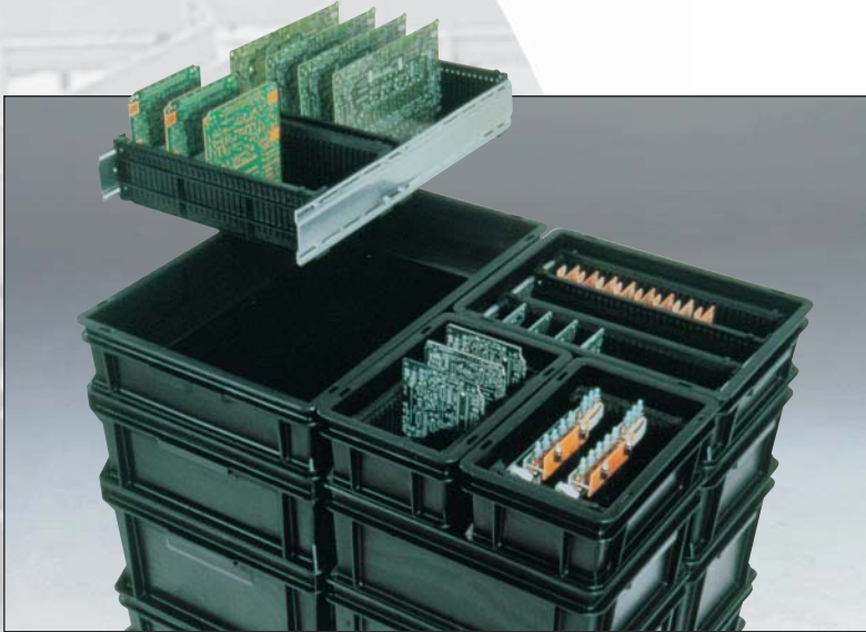
Behälter mit verstellbarem Einsatz für den Transport von Platinen. Beide sind aus ESD-sicherem (geschützt vor elektrostatischen Entladungen) Kunststoff hergestellt.
